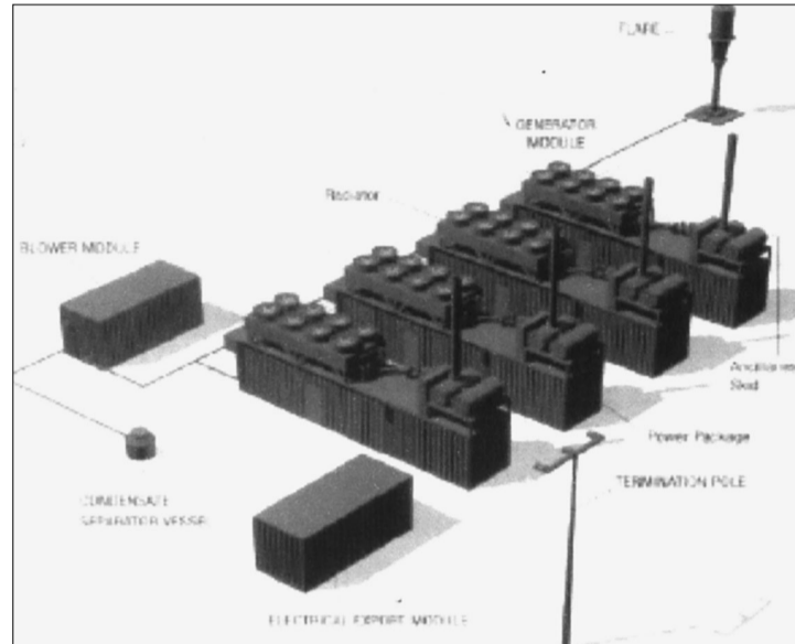
Μονάδα που χρησιμοποιεί τα αέρια της κατεργασίας των αποβλήτων (βιοαέριο) για την παραγωγή ηλεκτρισμού.
